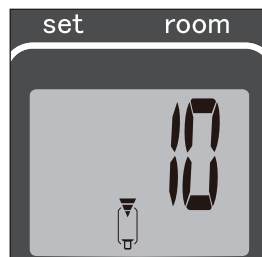
K: Cuando el indicador FUEL aparezca, la pantalla digital indicará los minutos restantes de combustible antes de que la estufa se apague.
