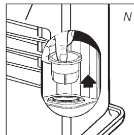
Brandstofzeefje
