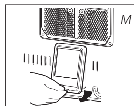
Polttoainesuodatin
